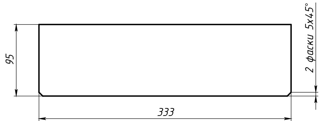
Поз.2 (Ребро)
